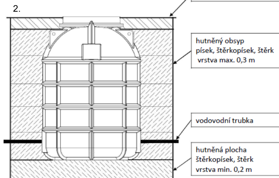
vzor - uložení bez přítomnosti podzemní vody
